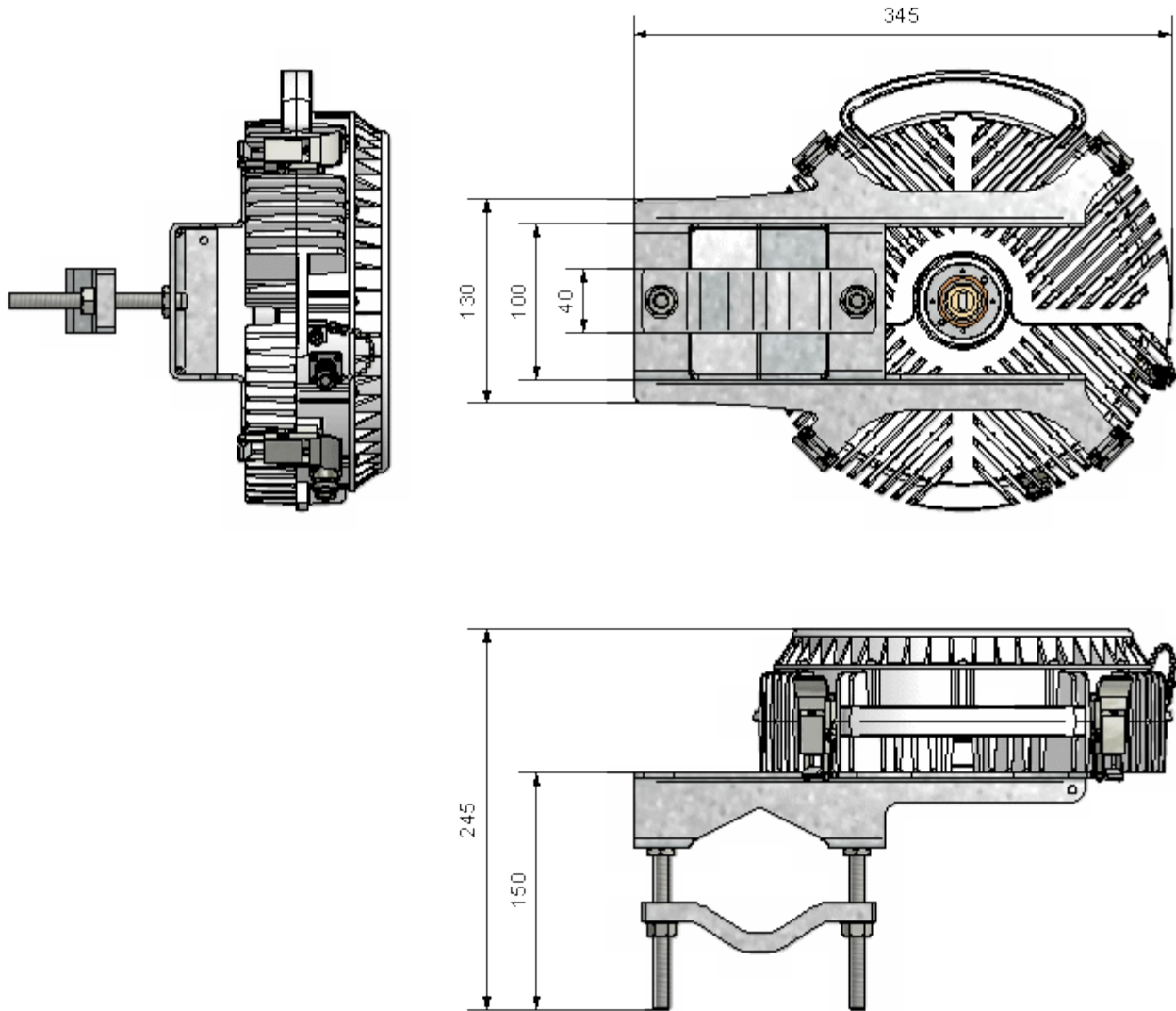
Obr. 7-2: Rozměry jednotky AL11F ODU s nosičem.
