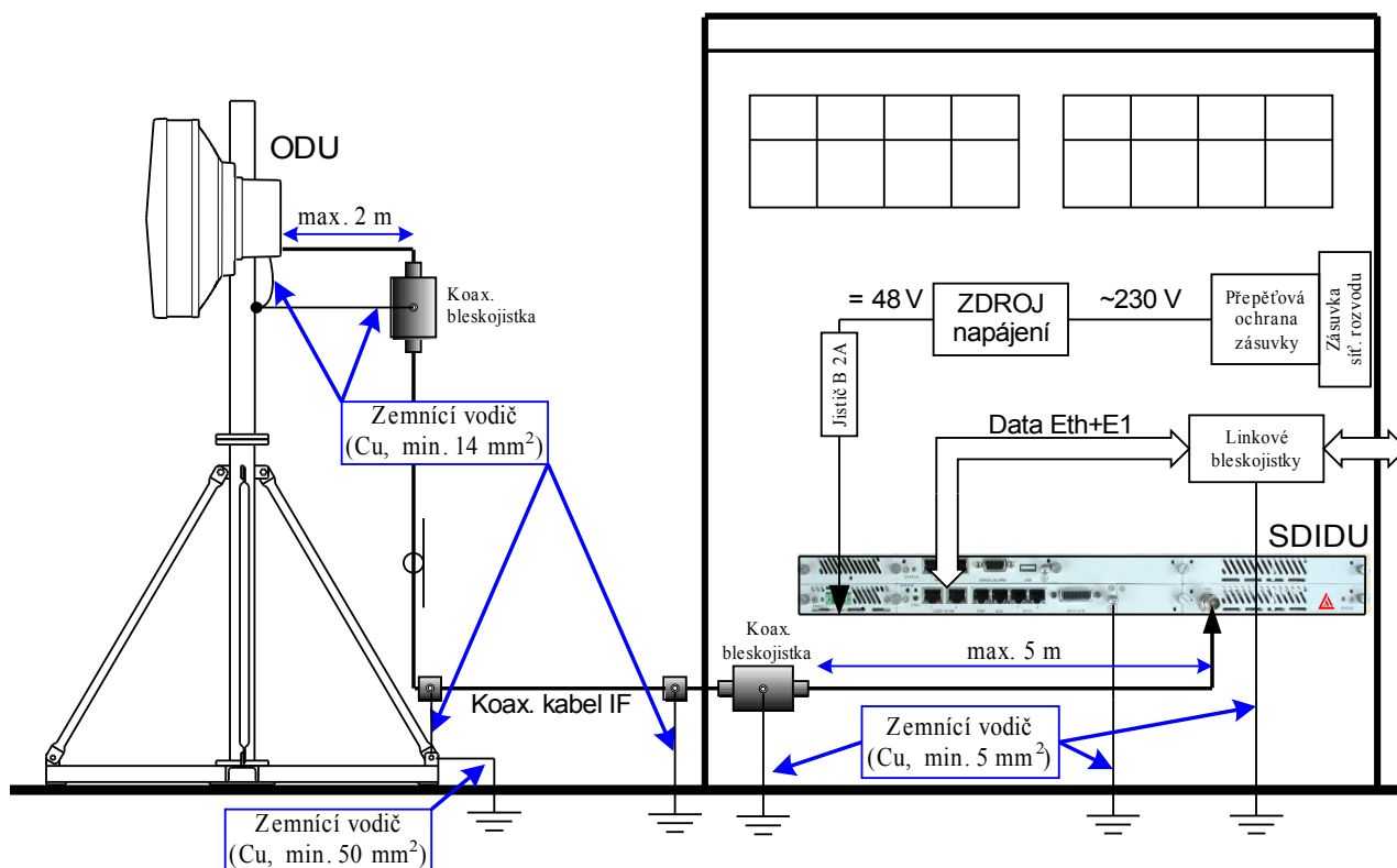
Obr. 4-2: Uzemnění terminálu
