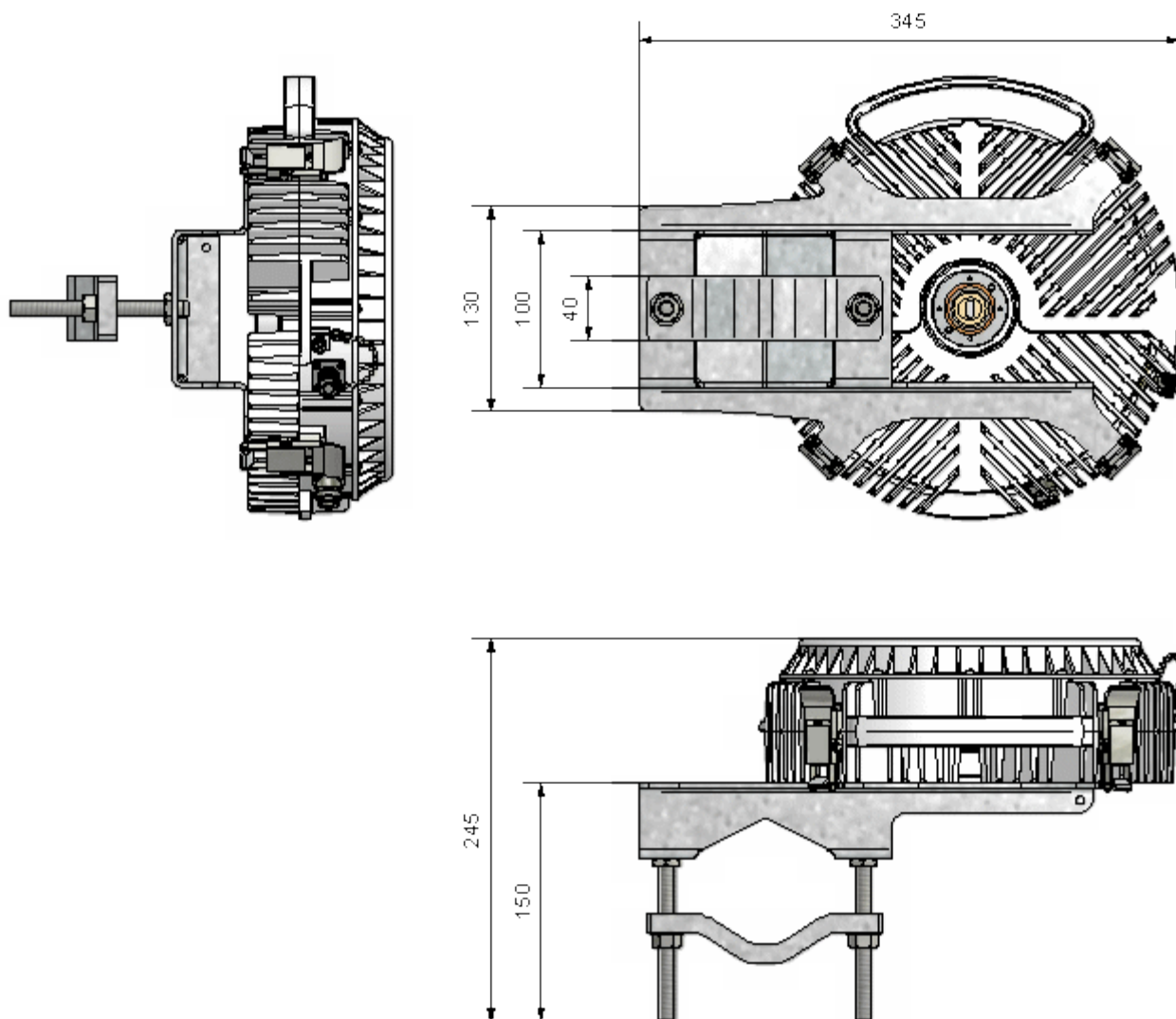
Obr. 7-2: Rozměry jednotky AL13F ODU s nosičem.
