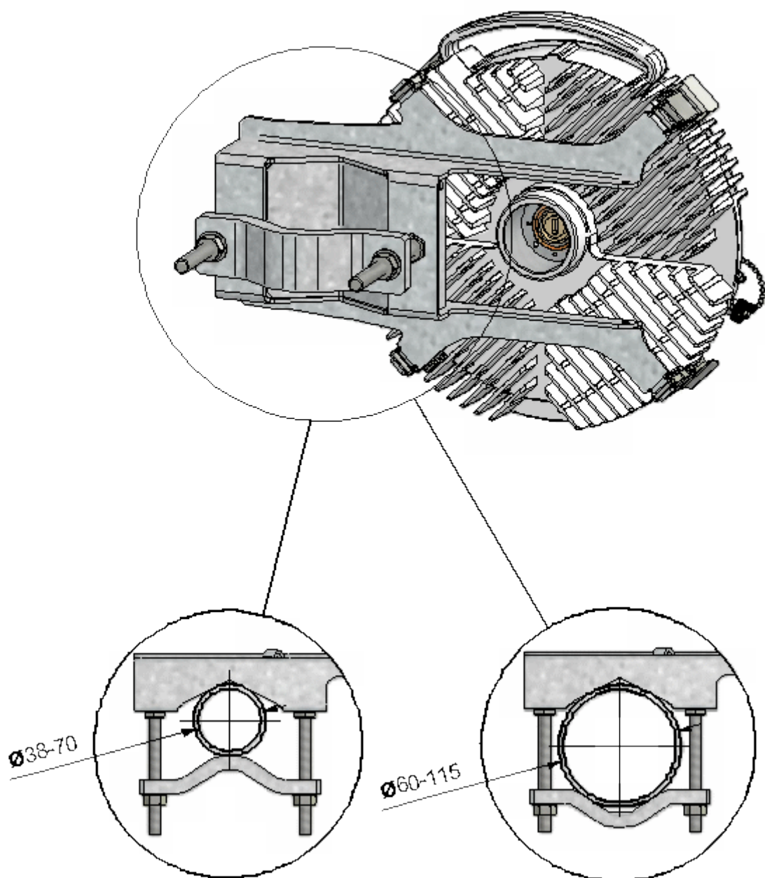
Obr. 7-3: Detail uchycení nosiče ODU ke stožáru.
