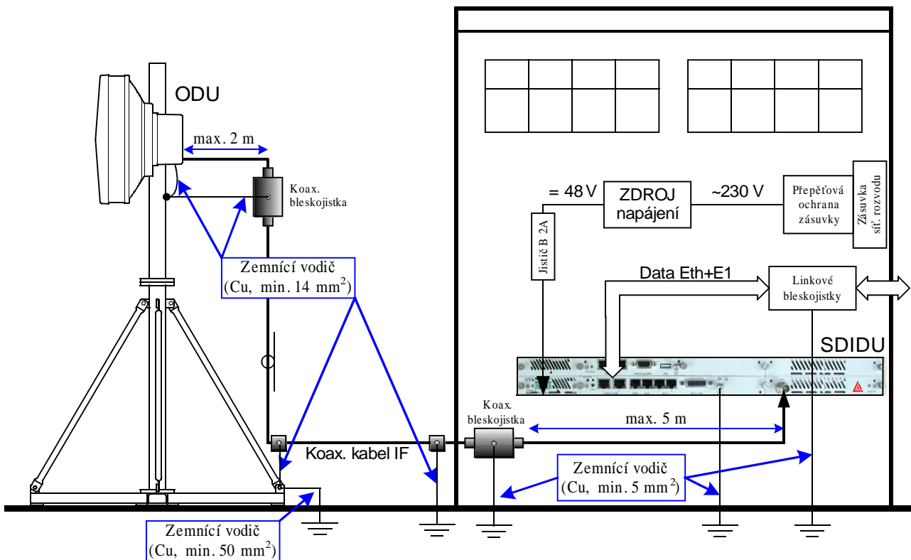
Obr. 4-2: Uzemnění terminálu
