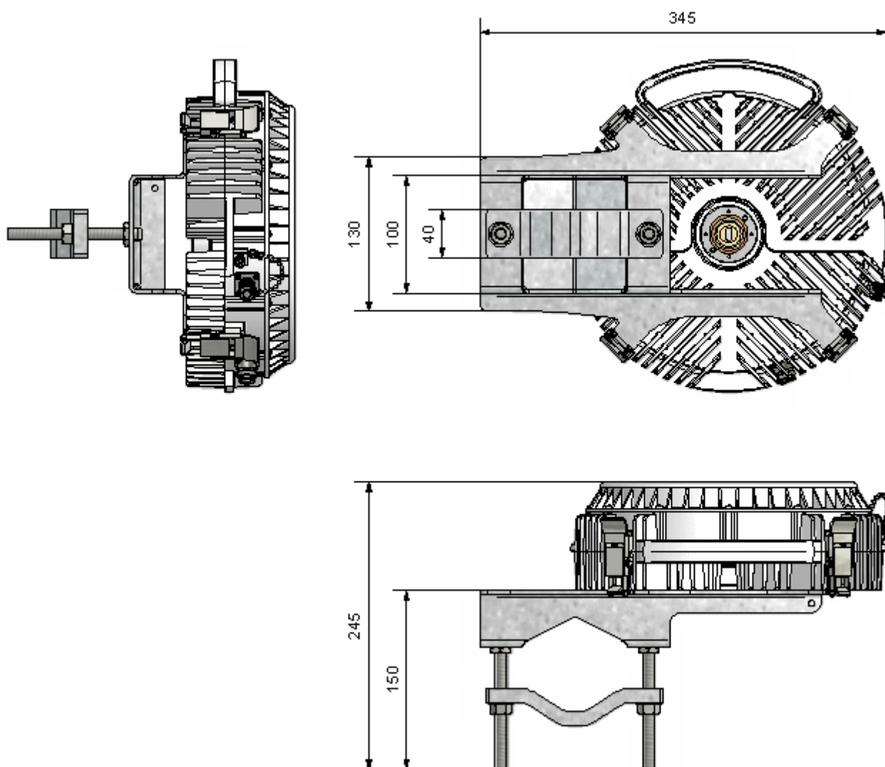
Obr. 7-2: Rozměry jednotky AL38F ODU s nosičem.
