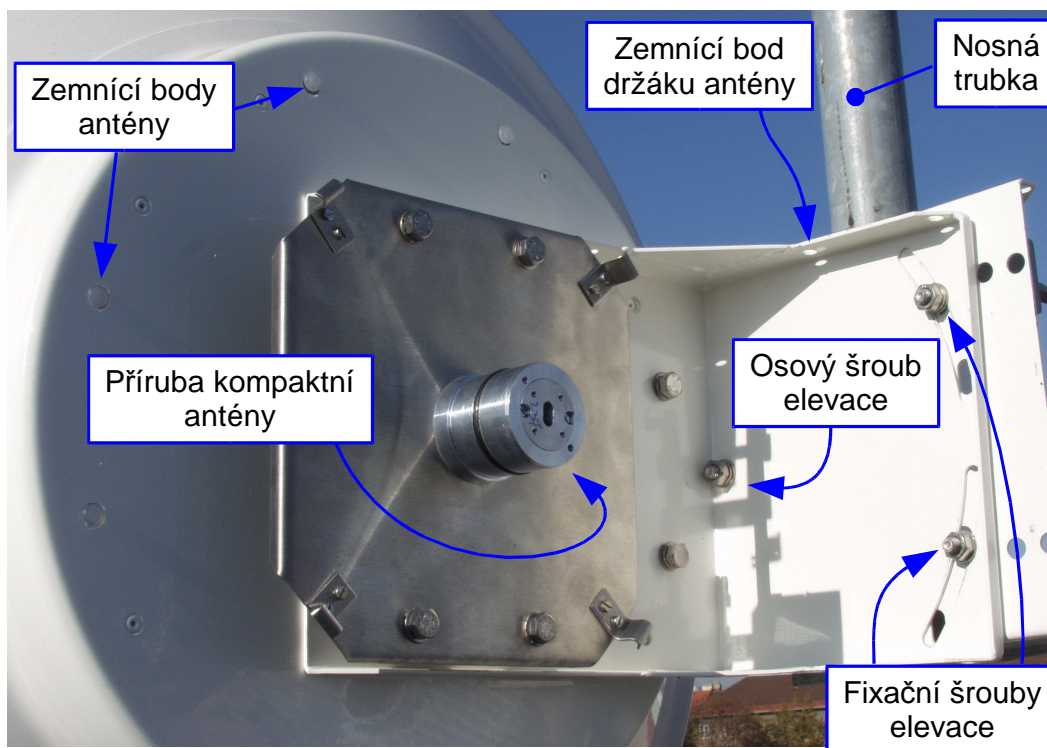
obr. 3-3: Instalace anténního systému
