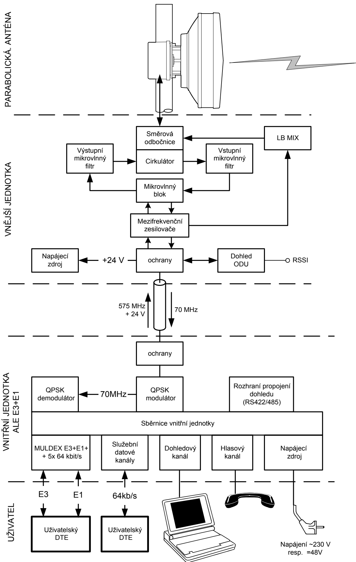
obr. 2: Blokové schéma stanice duplexního spoje AL18E E3+E1
