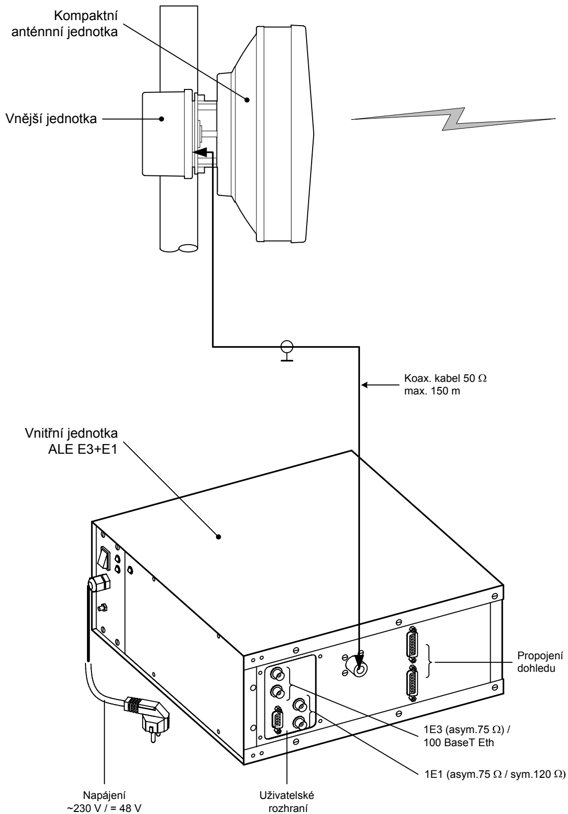
obr. 1: Uspořádání stanice mikrovlnného spoje AL18E E3+E1
