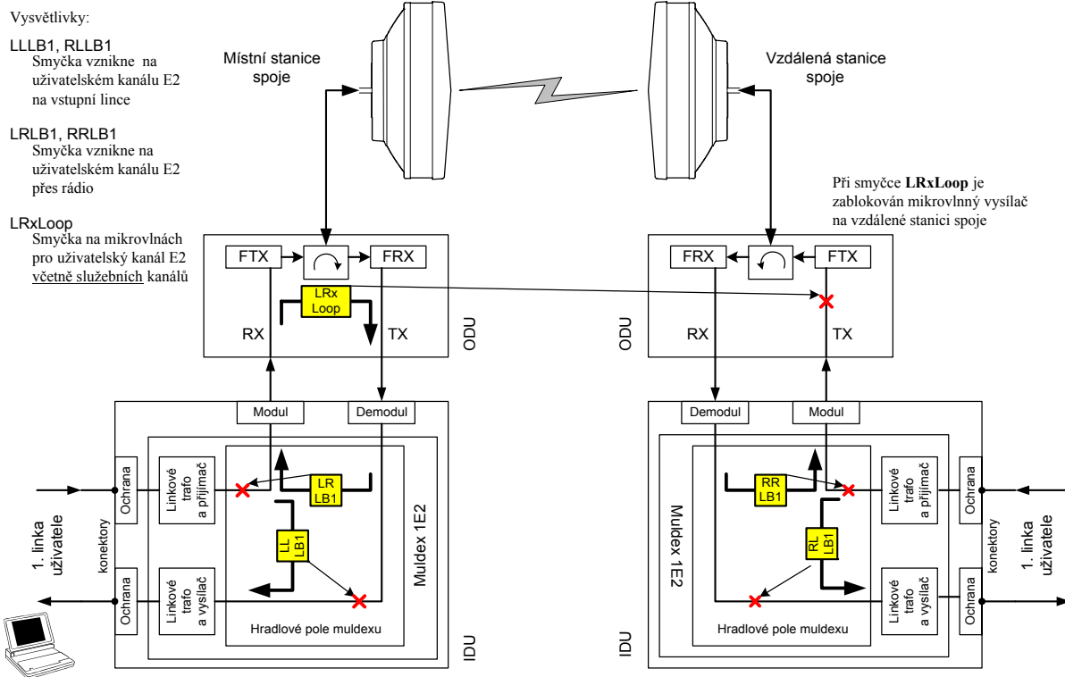
obr. 11: Měřicí smyčka na spoji AL18D 1E2
