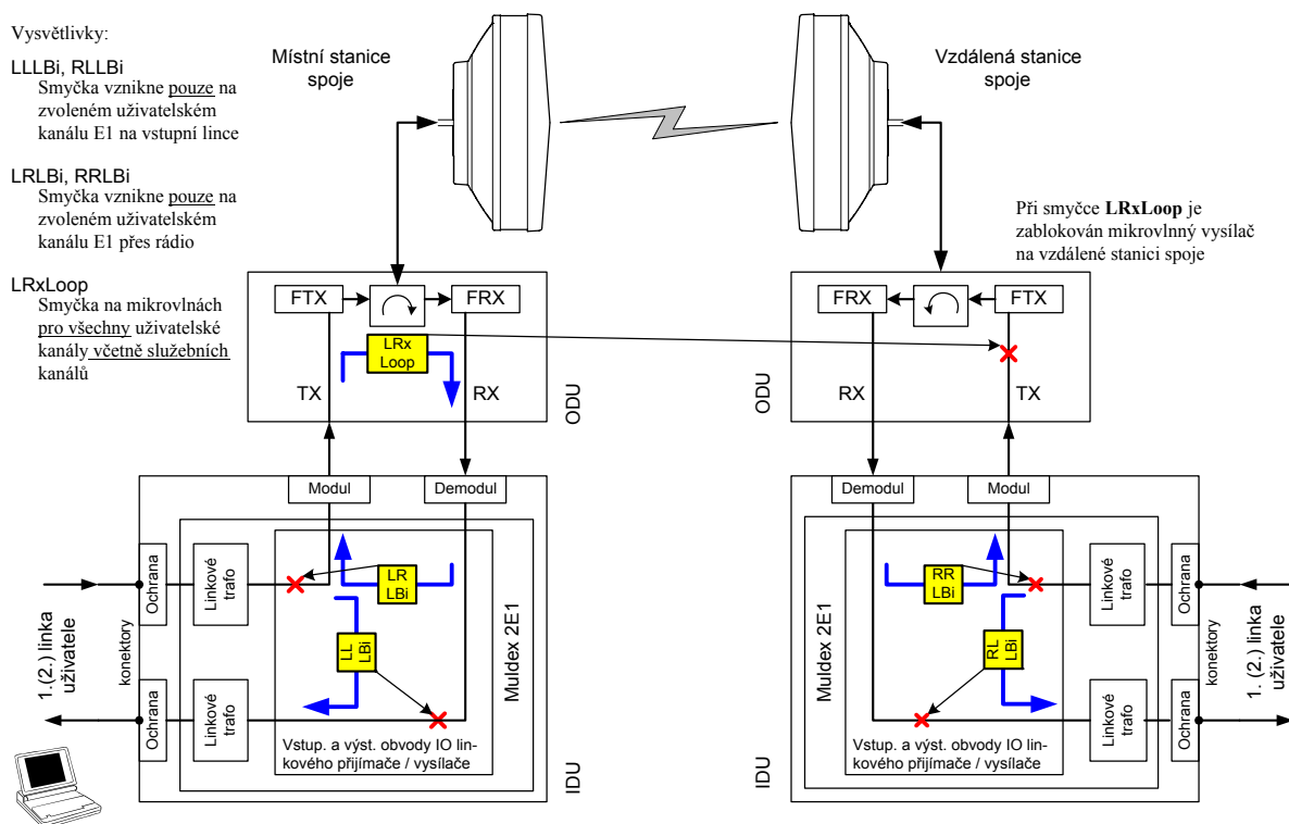
obr. 10: Měřicí smyčky na spoji AL18D 2E1
