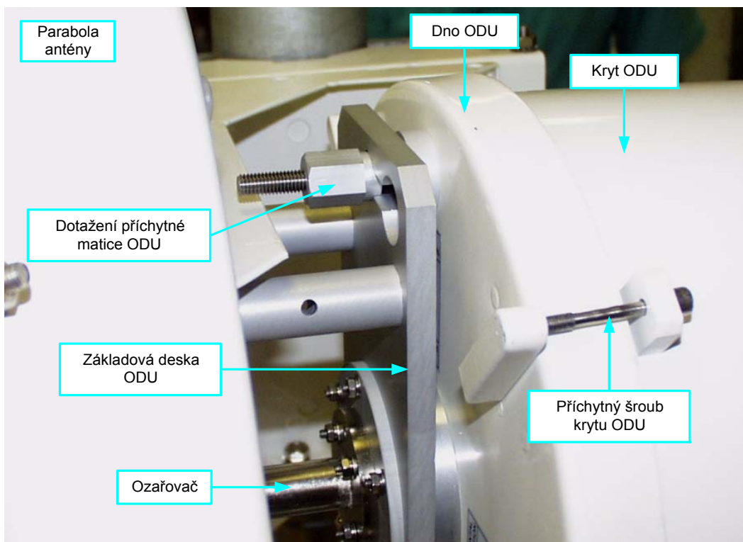
obr. 4: Uchycení ODU
