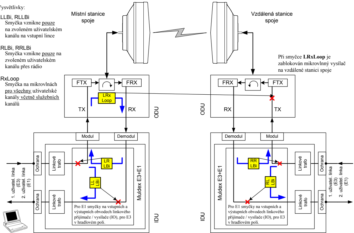
obr. 13: Měřicí smyčky na spoji AL18E E3+E1
