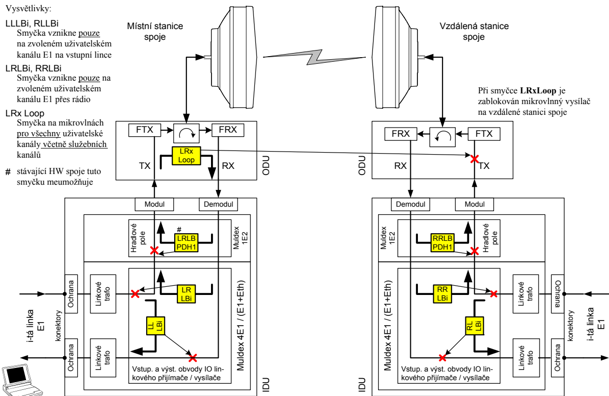
obr. 12: Měřicí smyčky na spoji AL18D 4E1, resp. AL18D Eth+E1
