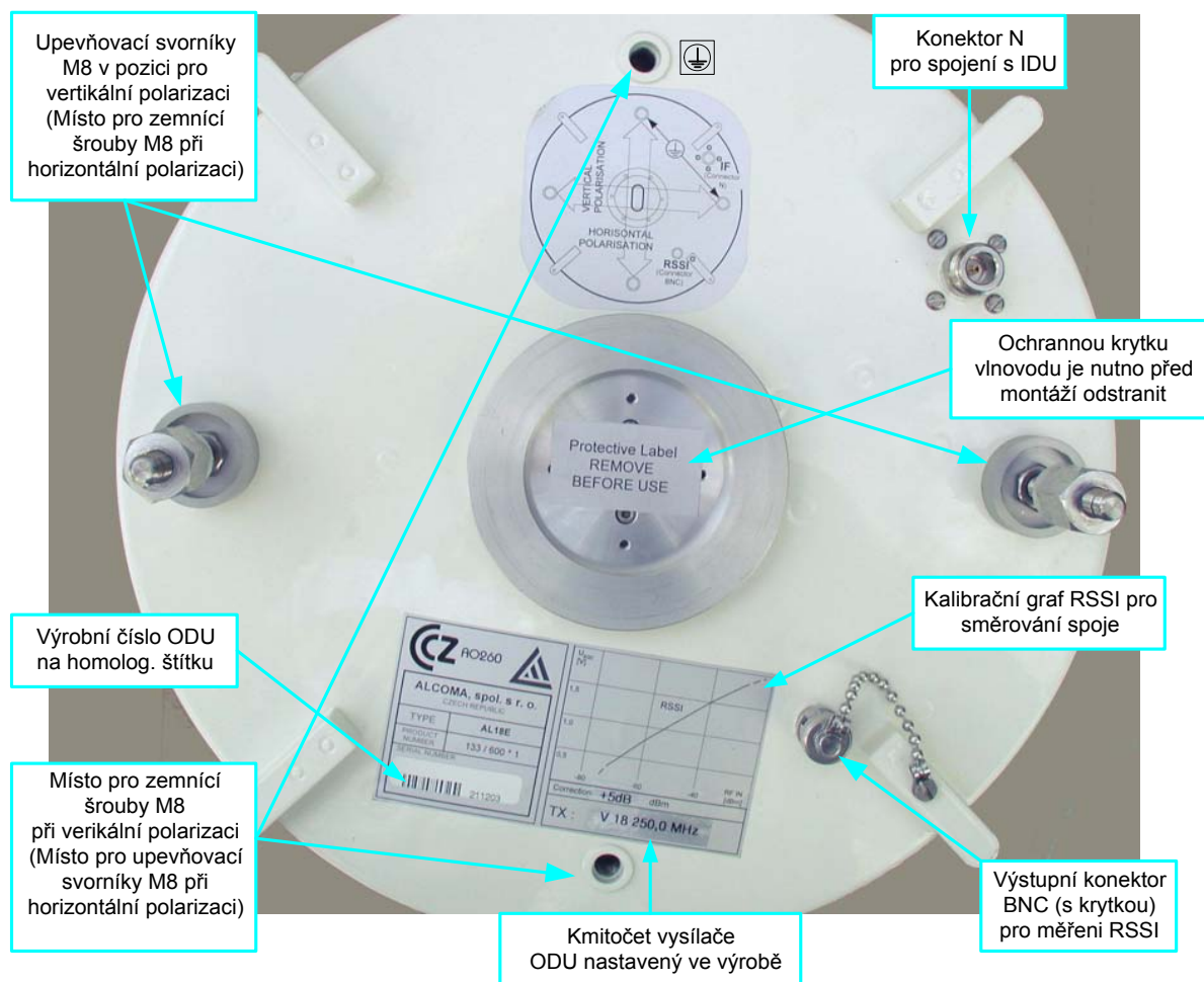
obr. 8: Poloha svorníků pro vertikální a horizontální polarizaci
