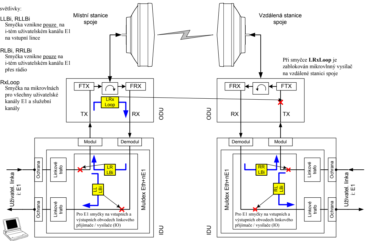
obr. 14: Měřicí smyčky na spoji AL18E Eth+E1 a AL18E Eth+nE1
